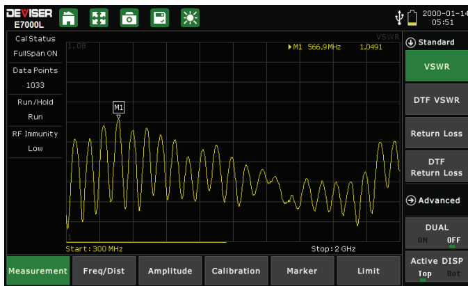
VSWR
