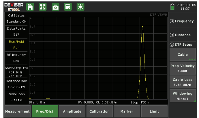
DTF-VSWR
